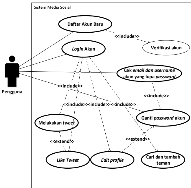
Gambar 3 Use Case Sistem
