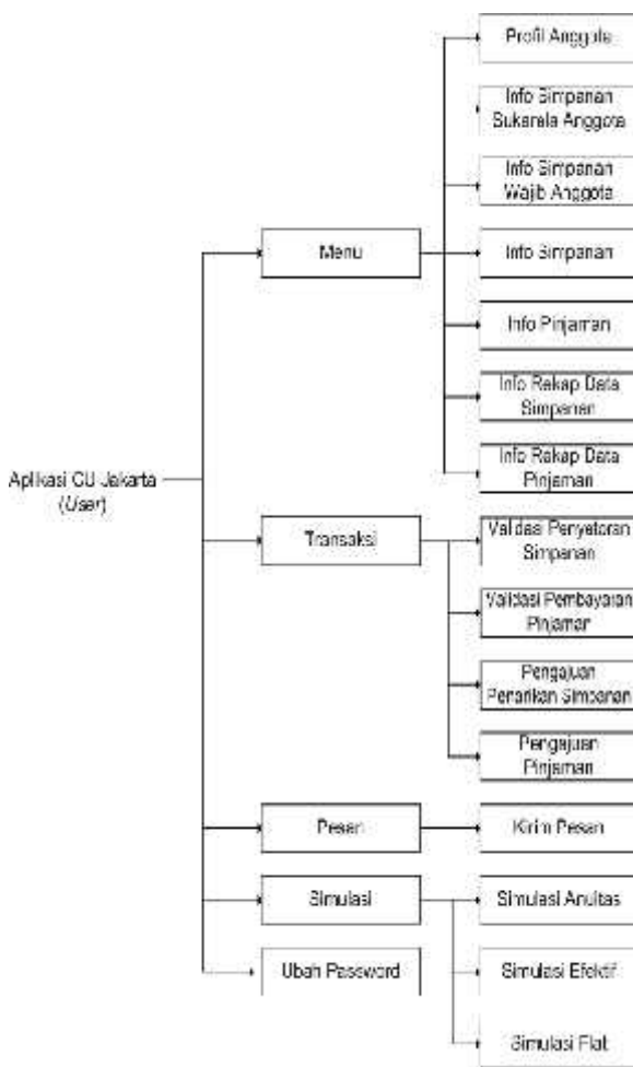
Gambar 4.2. Menu front-end
