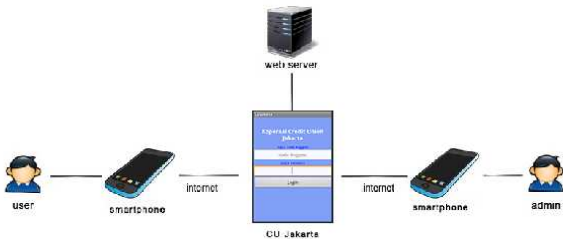
Gambar 4.1. Rancangan Arsitektur Sistem
