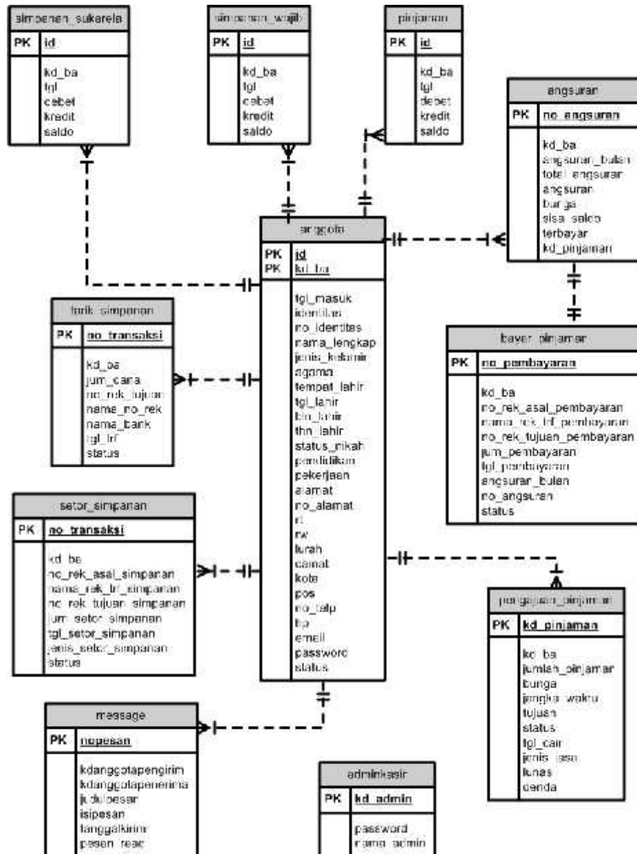
Gambar 4.4. ERD
